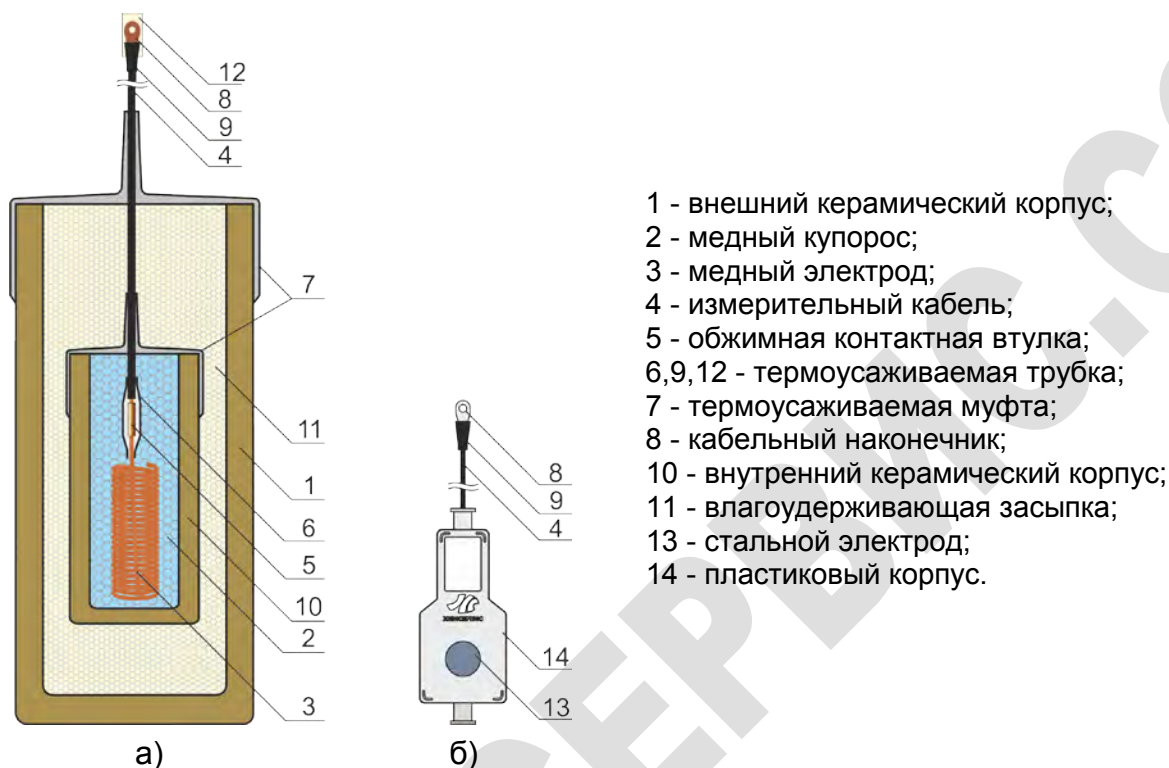
Рисунок 1 – Конструкция электродов:
