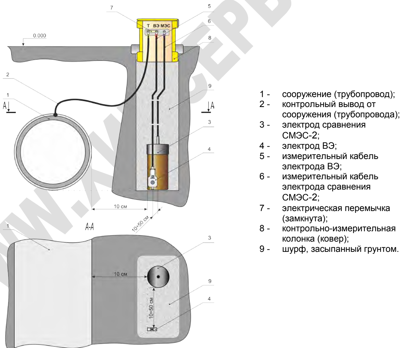
Рисунок 4 - Схема установки электродов
