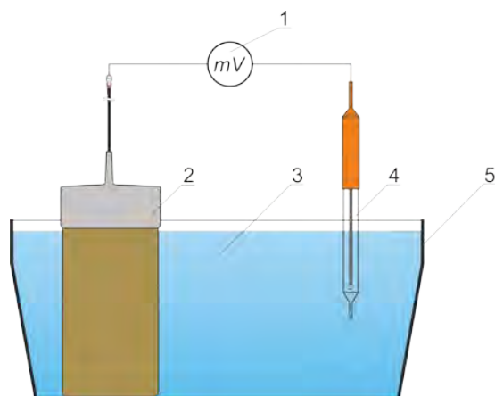
Рисунок А1 – Установка для измерения потенциала
