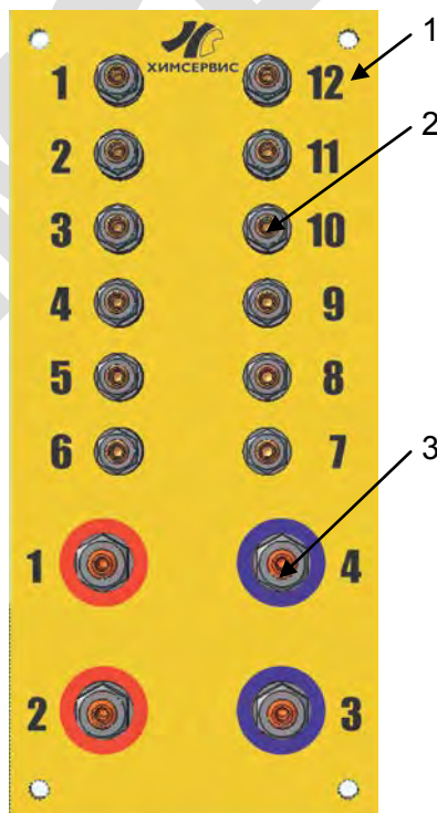
Рисунок А2 – Клеммная панель (исполнение 12-4) с клеммами
