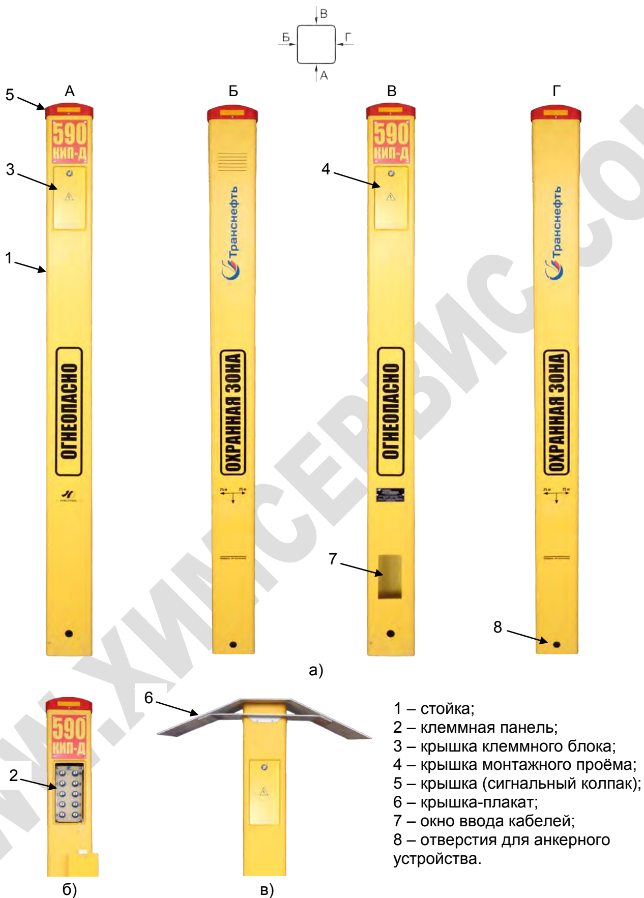
Рисунок 1 – Вид контрольно-измерительного пункта КИП ХС.ТН
