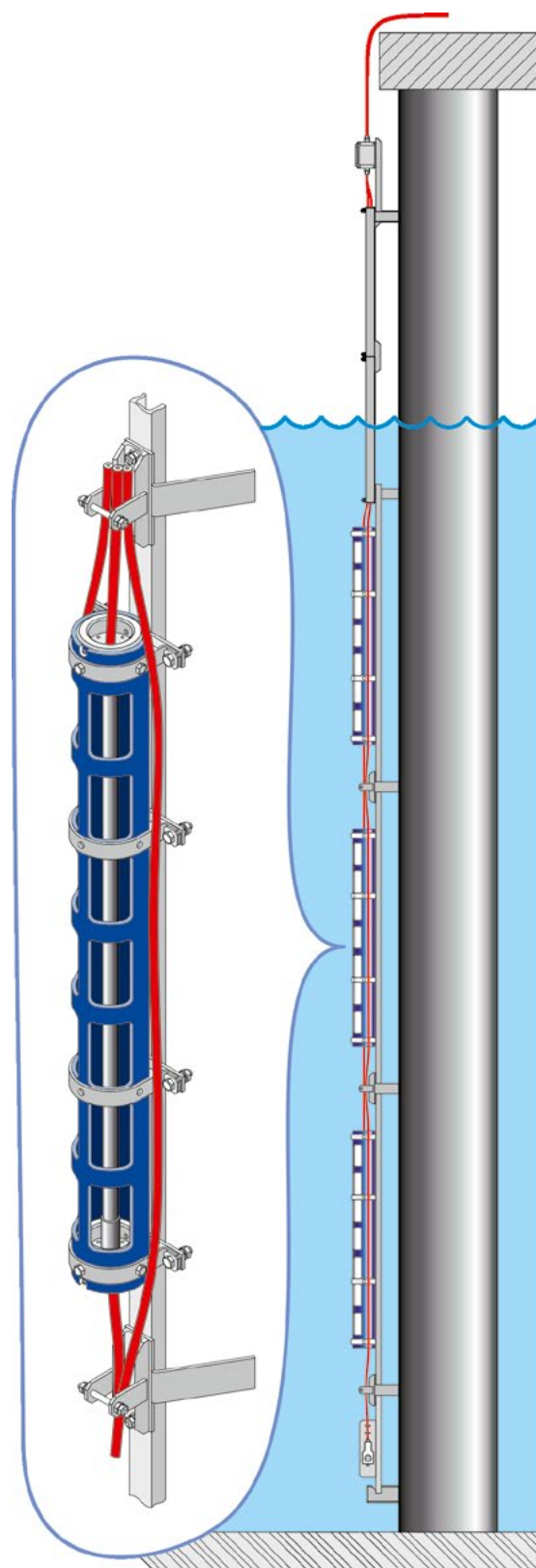
Свайная конструкция для установки подводных анодов на сваях причального сооружения
