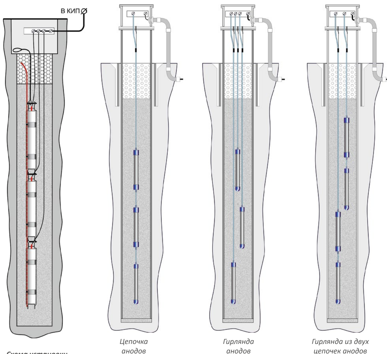
Схема установки глубинных магнетитовых или малорастворимых анодов
