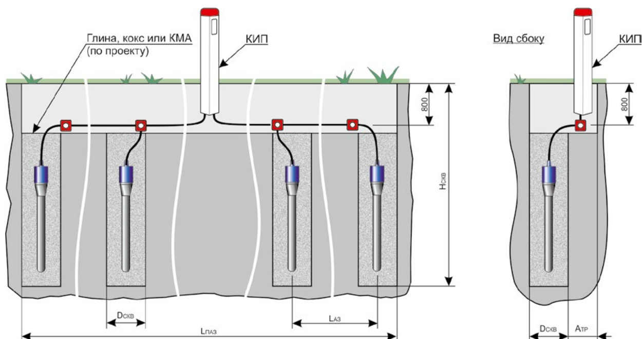
Схема горизонтальной установки подповерхностных анодов (в траншее)
